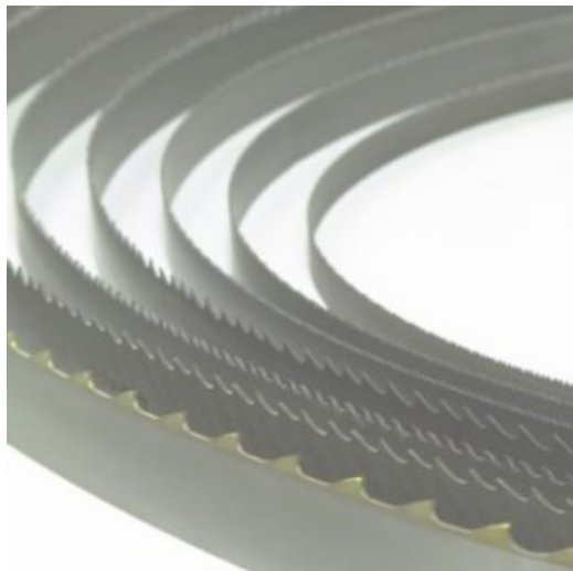
ЛЕНТОЧНЫЕ ПОЛОТНА Полотно ленточное М42 27/0,9/2460 ш.6/10 БИМЕТ
